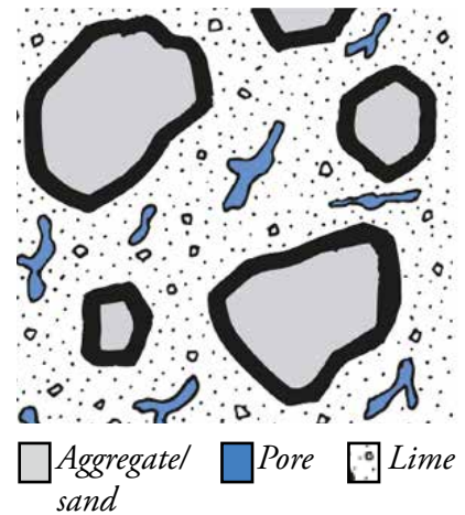
Mortar 1:1.
